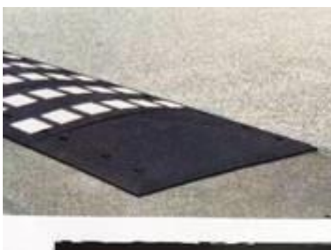
6-23501 Safety Rider venstre element. Typegodkendt fartdæmper der dæmper >40km/t. inkl skruer. Overkørselslængde: 90cm bredde/enhed: 50cm højde: 5,0cm
